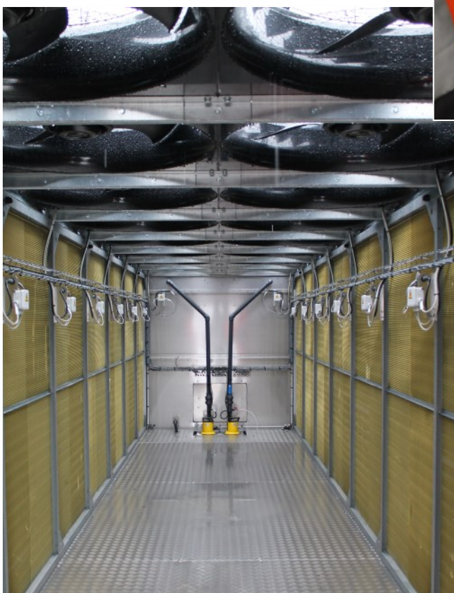
Condenseur adiabatique JACIR
