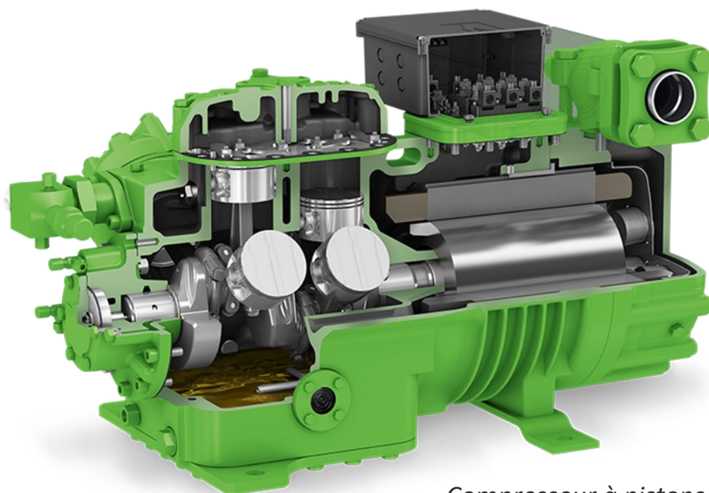
Compresseur à pistons BITZER
